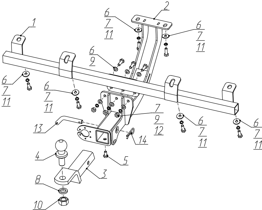
Схема монтажа
